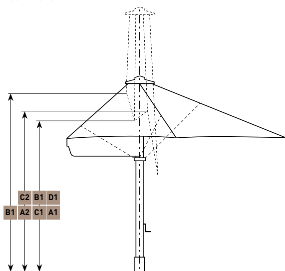
Seitenansicht A
